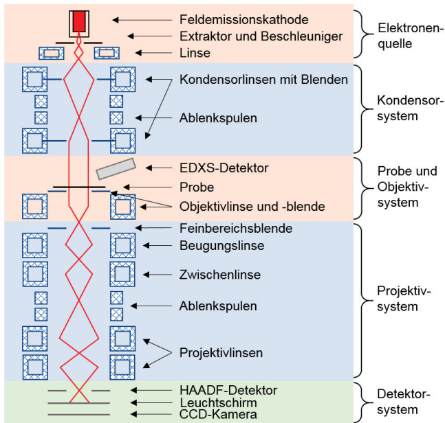
Abbildung 3. Schematischer Aufbau eines Transmissionselektronenmikroskops.
