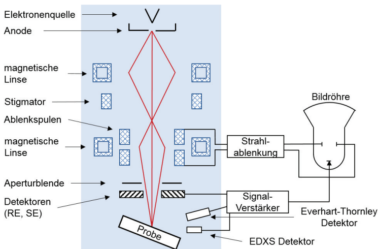
Abbildung 2. Schematischer Aufbau eines Rasterelektronenmikroskops.
