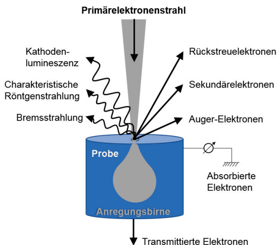
Abbildung 1. Schematische Darstellung der Wechselwirkung zwischen dem Primärelektronenstrahl und der Probe in einem Elektronenmikroskop (Abbildung modifiziert nach [44] ).
