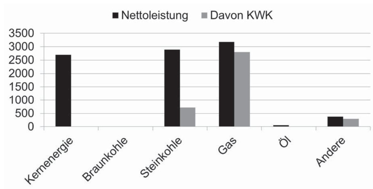
Abbildung 3: Niedersächsischer, konventioneller Kraftwerkspark mit Anteil an KWK-fähigen Kraftwerken über 100 MW (Datenquelle: [BNetzA 2016])
