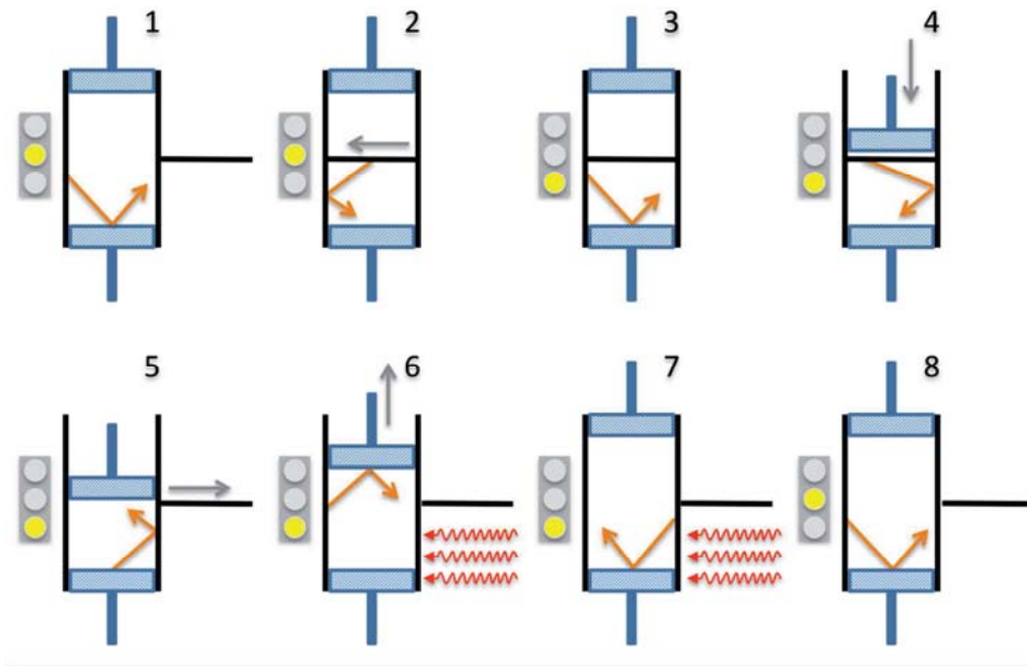
Abb. 3 Szilárds Modifikation von Maxwells Dämon
